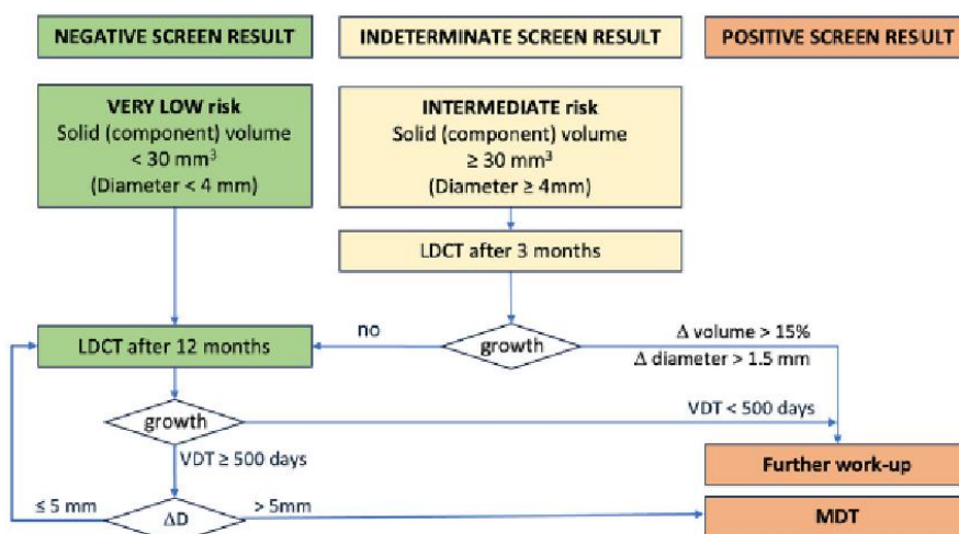
Figure 2 – Algorithme de gestion des nodules découverts lors d'un dépistage selon l'ESTI pour les nodules incidents. Extrait de (20)
